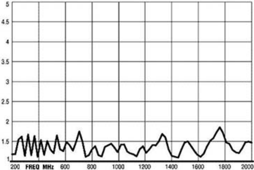
3148B Log Periodic Dipole Array Antenna VSWR
